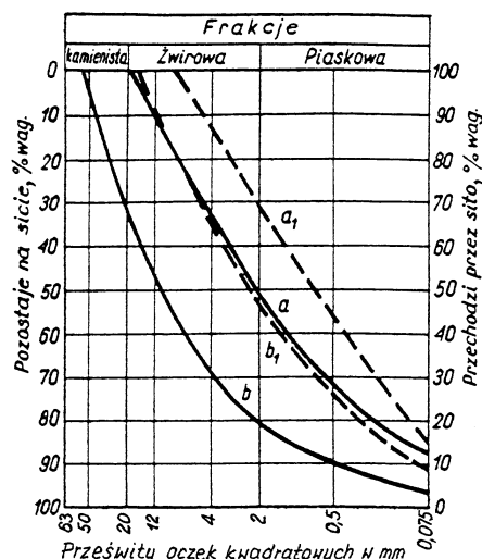
Rysunek 1. Obszar uziarnienia optymalnych mieszanek żwirowych
